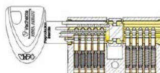
7101 VIP+ : cylindre profilé double / nickelé
