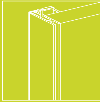
Crémaillère d'extrémité électrifiée avec panneau de 19 mm / Electrified lateral slot channel with 19mm panel
