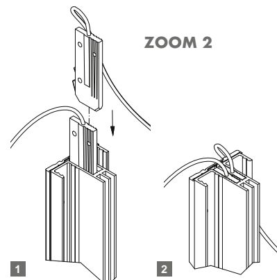
Sur crémaillière double Double-slot channel
