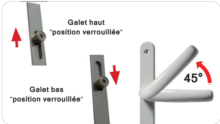
Relevage de la béquille
