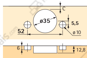
Cotes de perçage TH FIX
