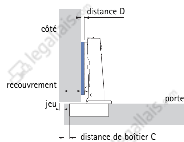
Cotes de perçage T FIX
