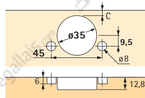
Cotes de perçage TB FIX
