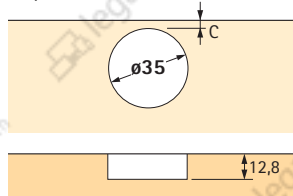
Cotes de perçage T FIX
