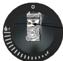
Vis de réglage Débit réduit (By-pass)
