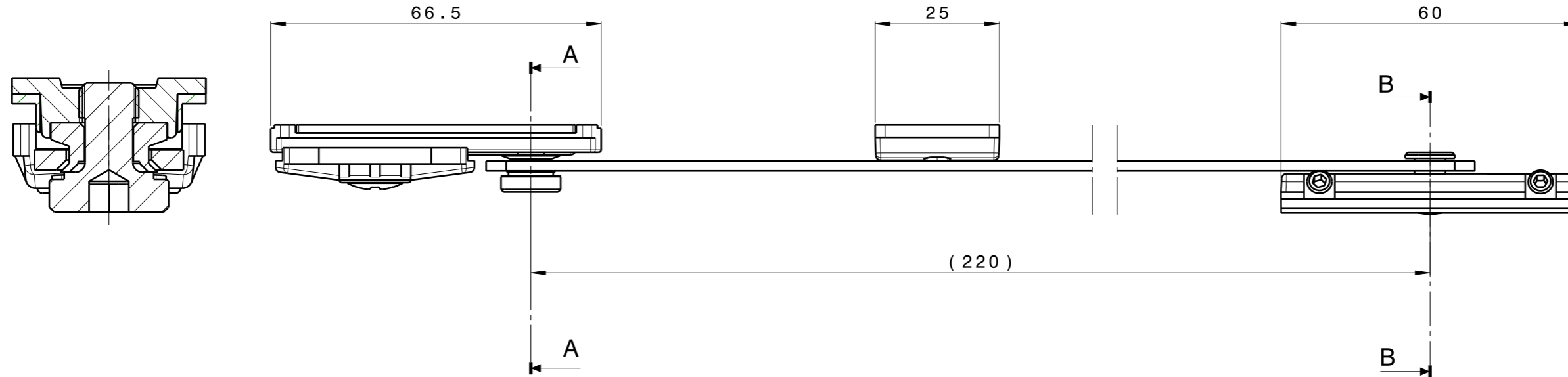
Vista in sezione A-A
