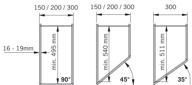
Aufansicht/Top view
