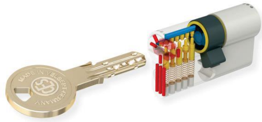
Cylindre WSM5 A2P1* brevet 2030, 4 clés
