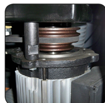
Toupie avec 3 vitesses de rotation Frees met 3 rotatiesnelheden
