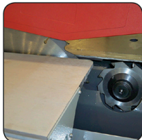
Lame ø 250 mm et inciseur ø 80 mm Blad met ø 250 mm en voorritser met ø 80 mm
