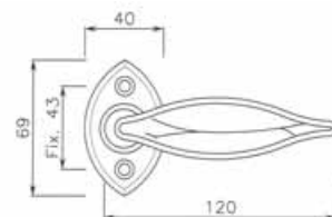
Béquille sur rosace LV102 Laiton vieilli Handle on LV102 rose Antique brass
