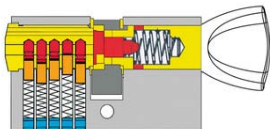
Cylindre à bouton
