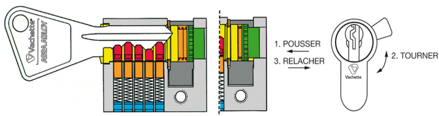
Demi cylindre
