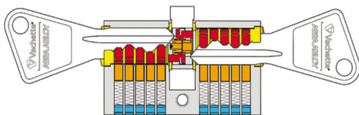
Cylindre double entrées SYNKRO
