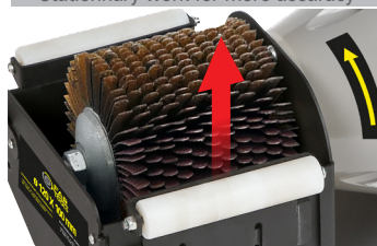
Rouleau d'appui réglable Adjustable tool support
