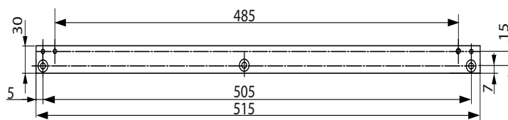
Plaque de montage plate A115 Pour bras à glissière G461.
