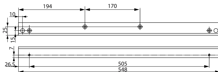
Support équerre A116 Pour installation côté opposé aux paumelles avec bras à glissière G461.
