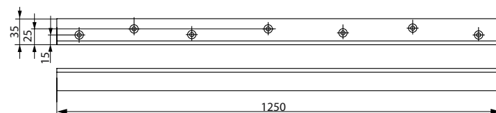
Support équerre A117 Support intermédiaire pour installation côté opposé aux paumelles avec bras à glissière G461.
