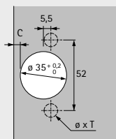
en applique (base B 12,5 mm)
