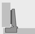
en applique (base B 12,5 mm)
