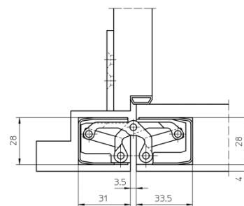
ébrasement chambranle
