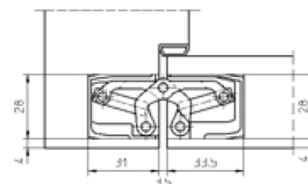
bloc-porte
