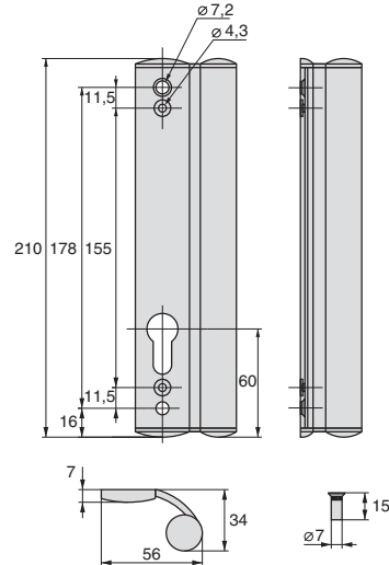
Poignée borgne 6408 Solid handle
