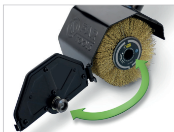
Changement rapide de brosse Quick brush change
