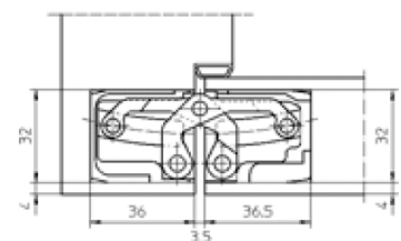
bloc-porte
