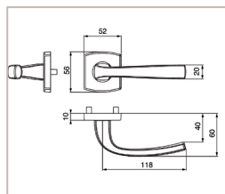
Ensemble sur rosace : réf 4075/6425
