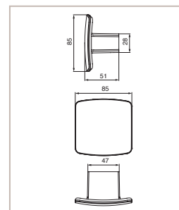
Bouton centre de porte : réf 5225
