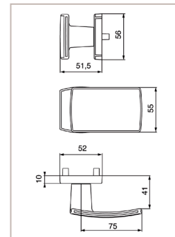
Palière sur rosace : réf 525/4075/6425
