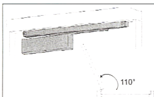
Montage sur la porte Côté à pousser
