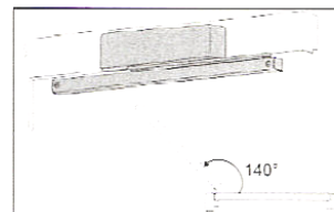
Montage renversé Côté à pousser - Dormant à fleur
