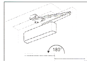
Montage bras parallèle
