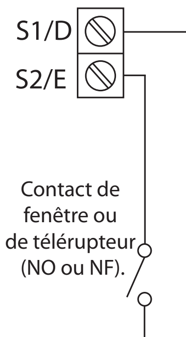
Configuration pour contact de fenêtre ou autre contact comme un télérupteur.
