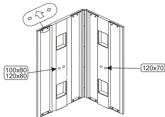
MONTAGE A DROITE/ RIGHT ASSEMBLING/ MONTAGE RECHTS
