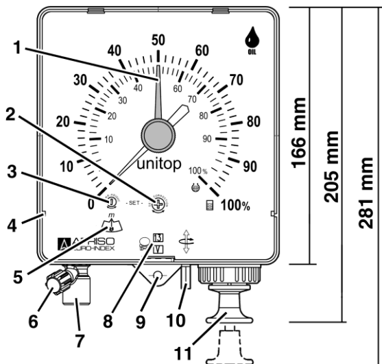
Figure 1 : Vue de face Unitop
