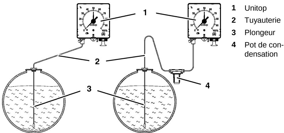
Figure 2: Unitop sans (gauche) ou avec (droite) pot de condensation
