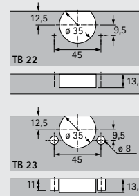
Schéma de perçage 45 x 9,5 mm
