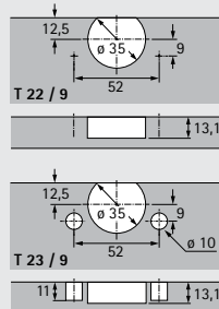
Schéma de perçage 52 x 9 mm
