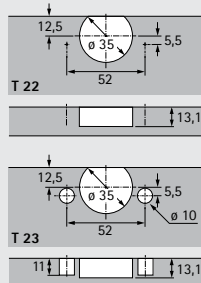
Schéma de perçage 52 x 5,5 mm
